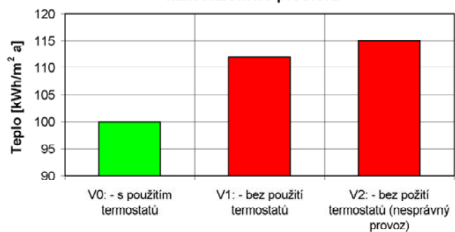
Spotřeba tepla na vytápění běžného kancelářského prostoru
