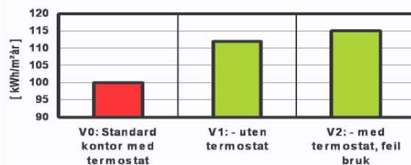
Energibruk oppvarming
